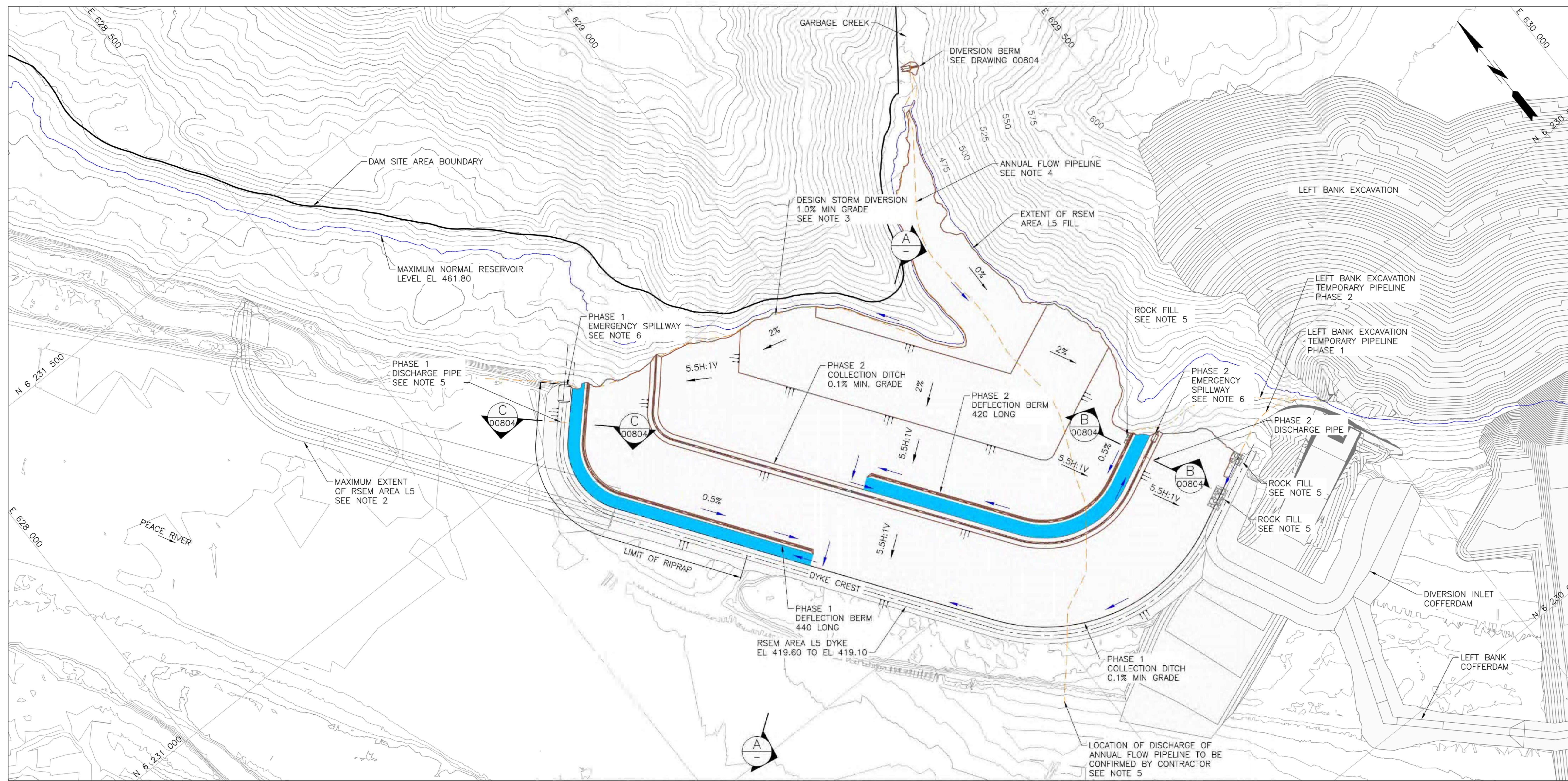
PLAN 1:2500
